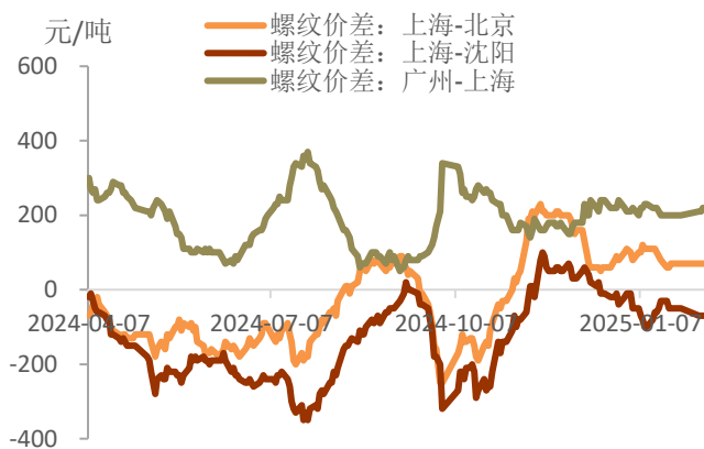
图表 5 螺纹钢现货地区价差走势
